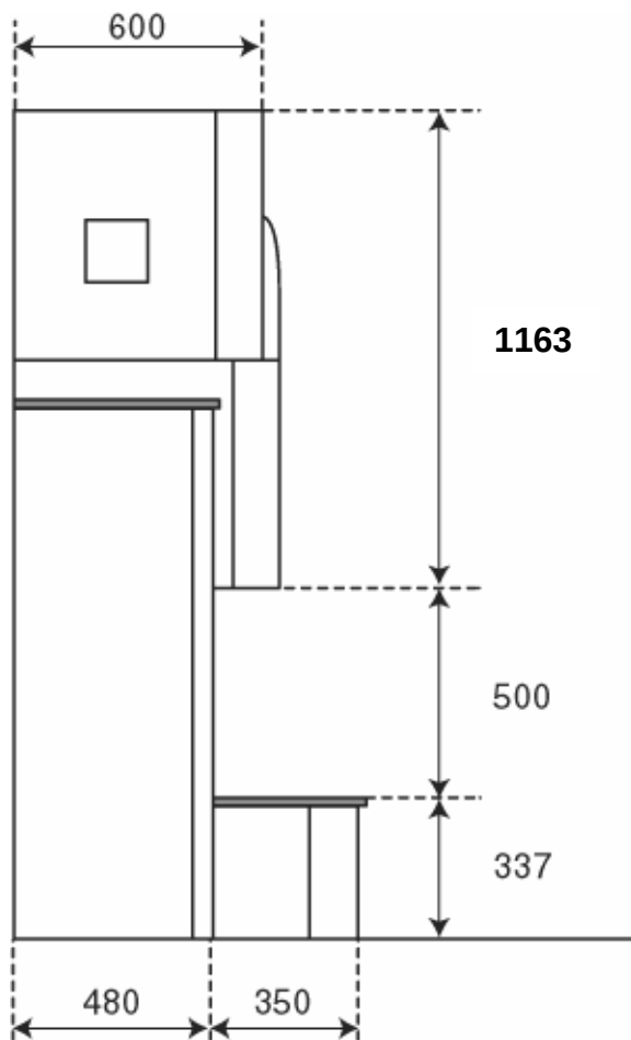
Abbildung 7: Abmessungen
