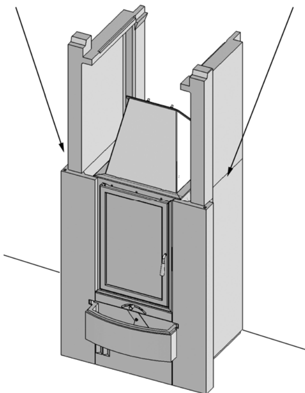
Abbildung 6 + 7: Montage der Kaminhaube links und rechts
