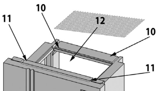
Abbildung 9: Montage der Auflager vorne und hinten sowie des Luftgitters
