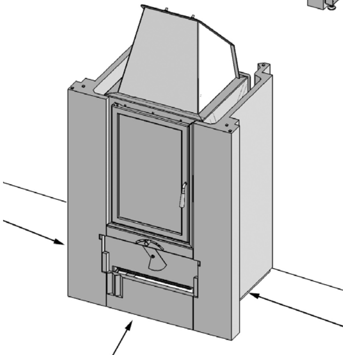
Abbildung 3: Montage der Seitenelemente und der Sockelplatte vorne
