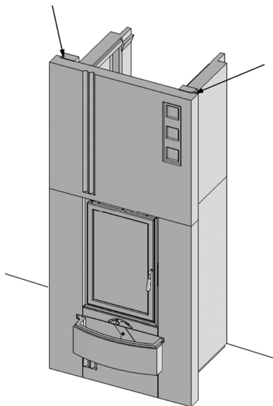
Abbildung 8: Montage der Kaminhaube vorne
