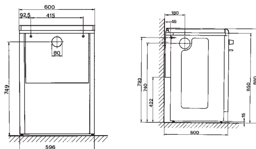
Abmessungen
