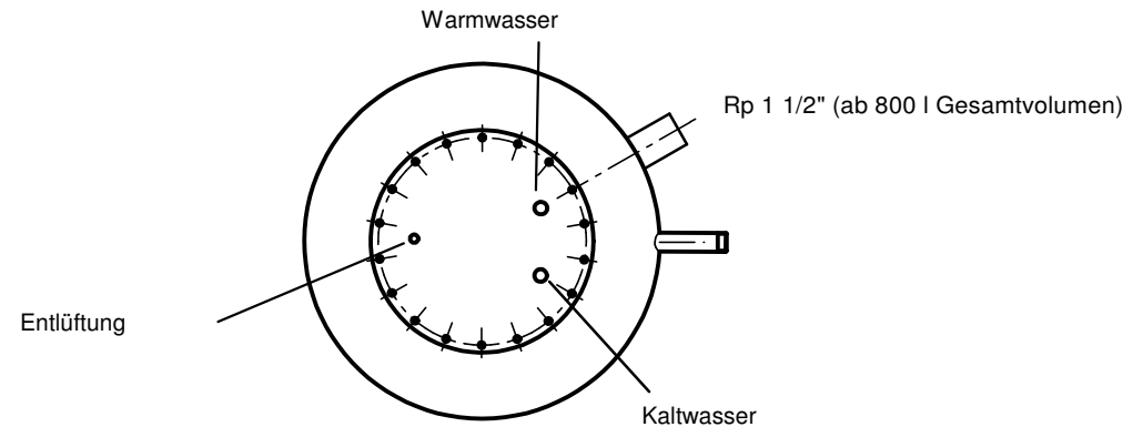
Behälteransicht von oben
