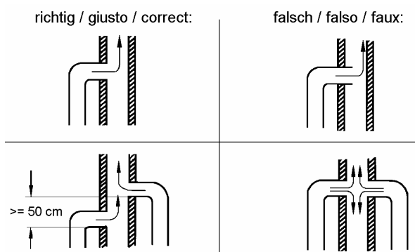
Abbildung 13: Rauchrohranschluß am Schornstein (Kamin, Rauchfang)
