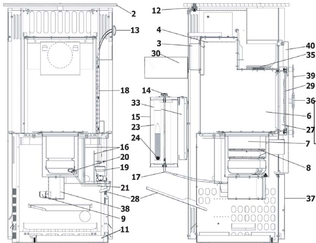
Abbildung 2: Ölofen Ibiza 469.50
