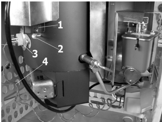
Abbildung 17: elektr. Zündung
